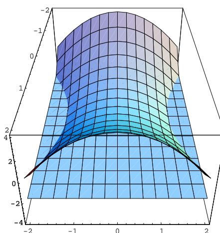
Intersezione col piano z = -2
