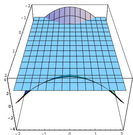
Intersezione col piano z = 2
