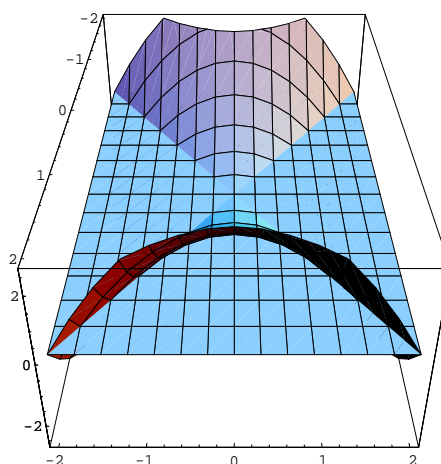
Paraboloide iperbolico: intersezione col piano z = 0
