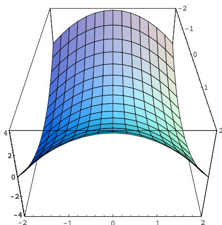
Paraboloide iperbolico: restrizione a [-2, 2] \times [-2, 2]
